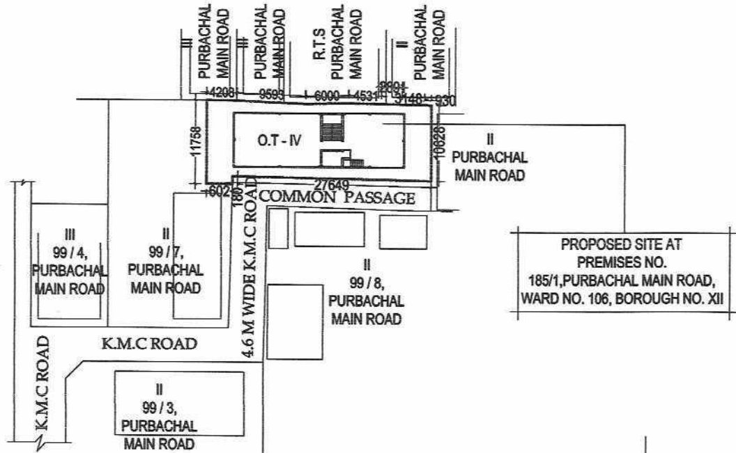
SITE PLAN SCALE - 1:600
